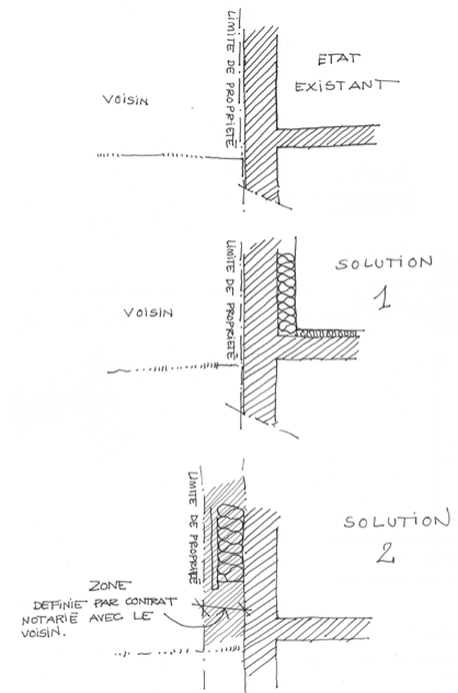
croquis réalisés lors d'un rendez-vous avec un particulier sur le thème : Isolation par l'extérieur en limite de propriété,
